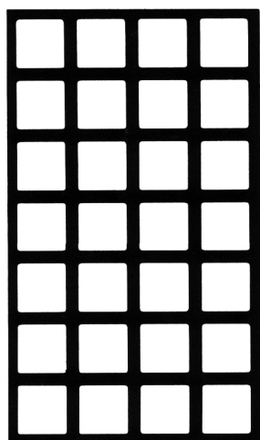
305 8□×10P 開孔率 64%
