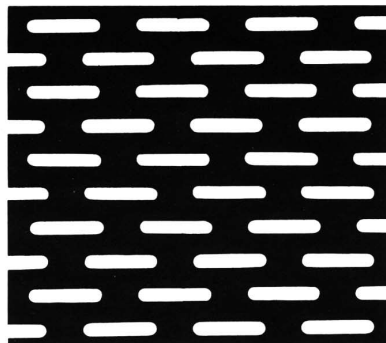
201 2×11 開孔率 27%
