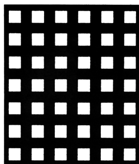
302 4□×7P 開孔率 32.7%
