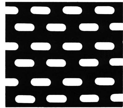
206 4×11 開孔率 29%
