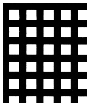
303 5□×8P 開孔率 39%
