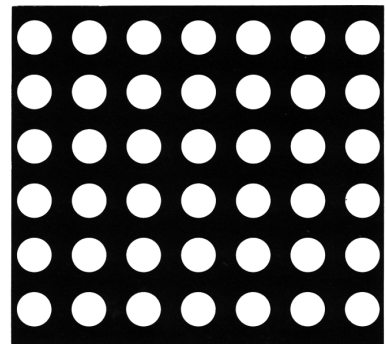
106 5\phi \times 8P 開孔率 30.7%
