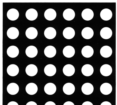
109 6\phi \times 9P 開孔率 35%
