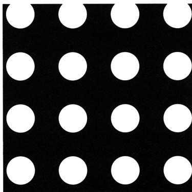
111 8\phi \times 15P 開孔率 22.3%
