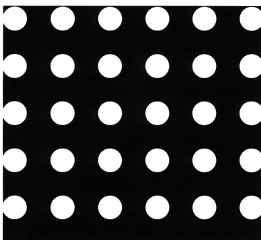
107 5\phi \times 10P 開孔率 19.6%
