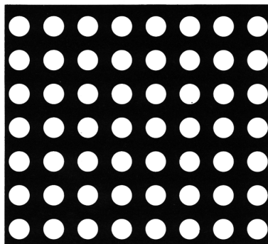
104 4\phi \times 7P 開孔率 25.6%
